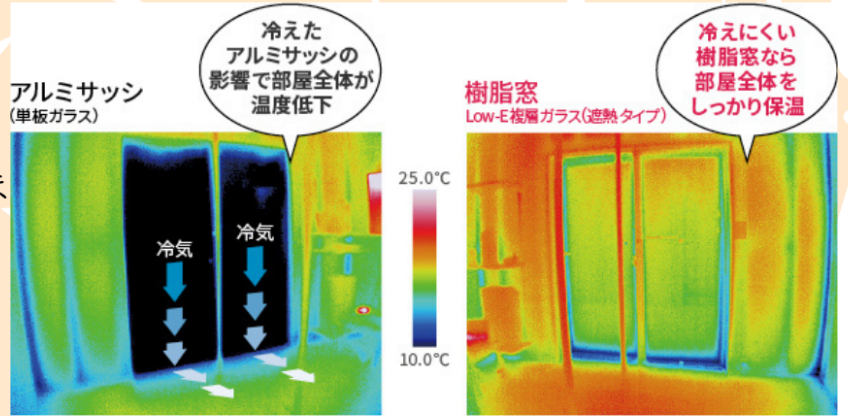
床暖房停止後4時間経過時をサーモグラフィカメラで撮影。社内試験による。
